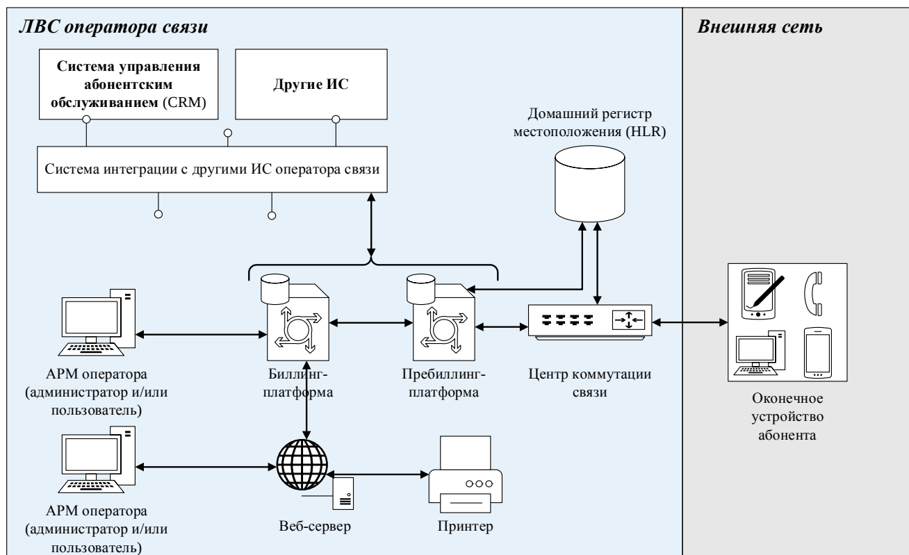
Рисунок 6 – Схема типовой автоматизированной системы расчетов
