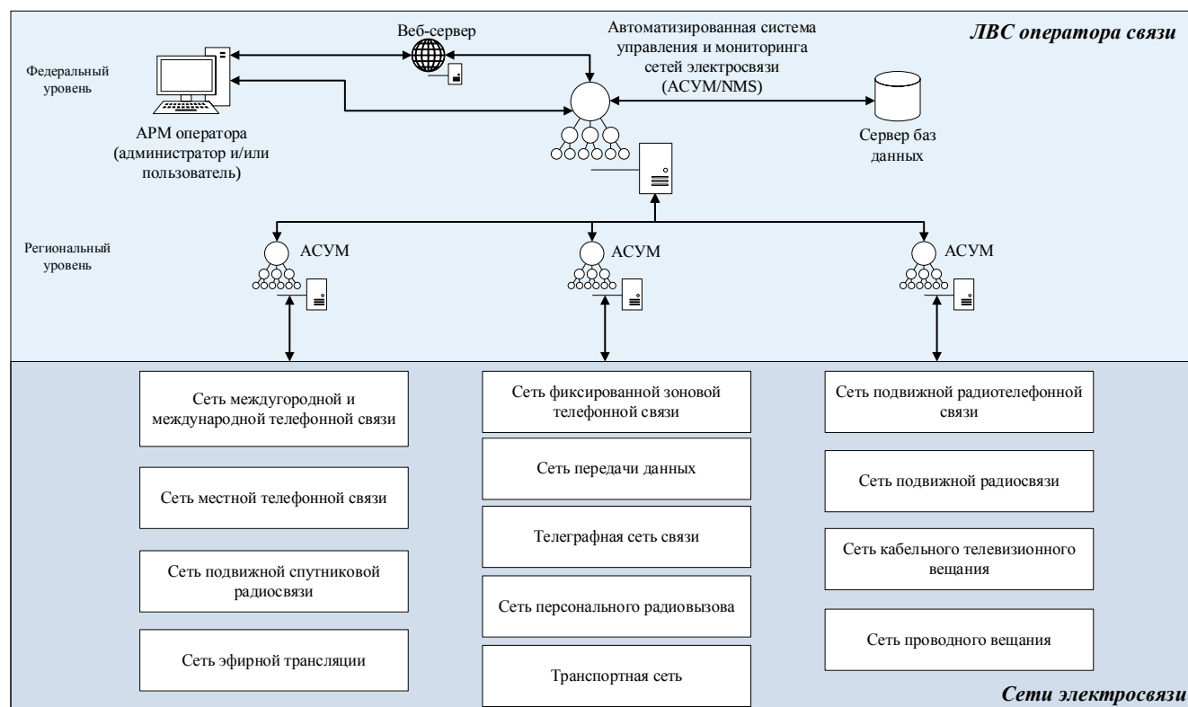
Рисунок 8 – Схема типовой автоматизированной системы управления и мониторинга сетей электросвязи
