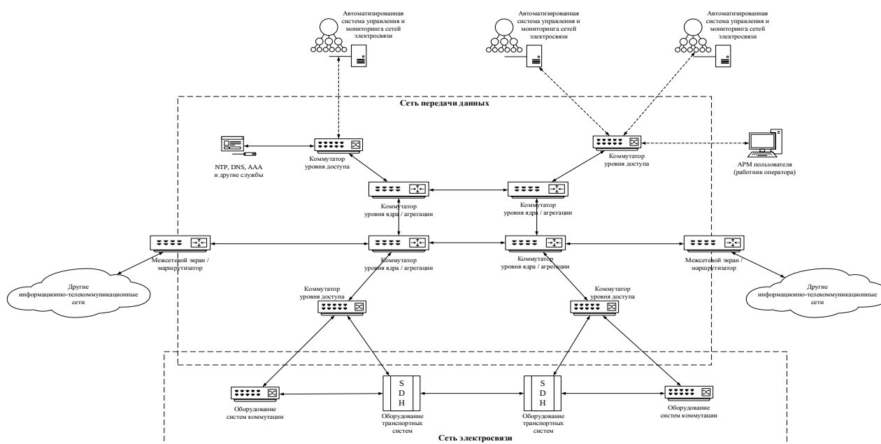
Рисунок 10 – Схема типовой выделенной сети передачи данных для управления и мониторинга сетей электросвязи
