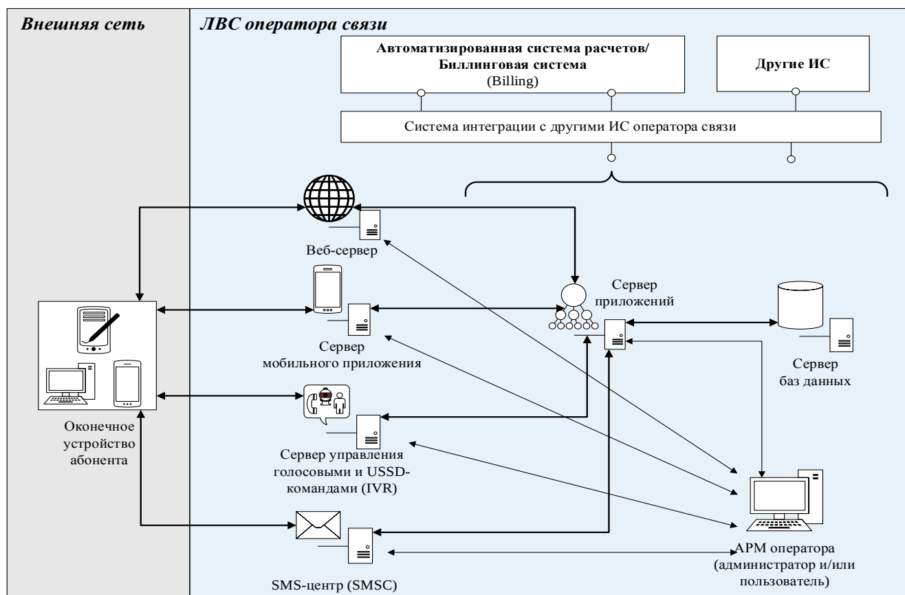
Рисунок 7 – Схема типовой системы самообслуживания абонентов
