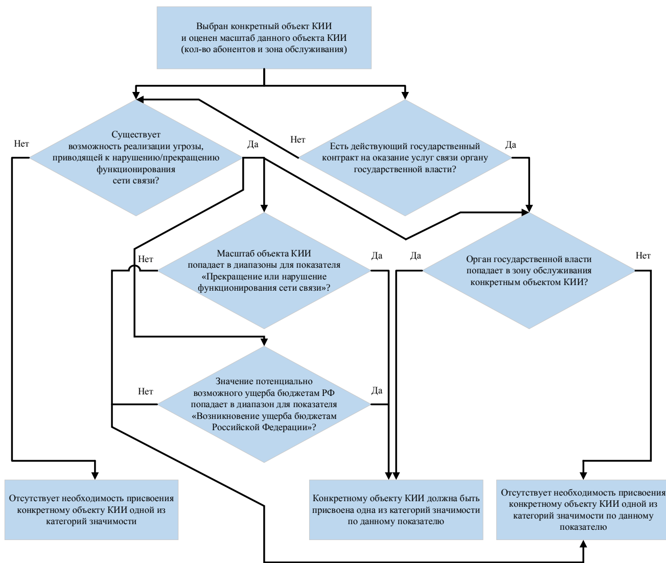
Рисунок 5 – Блок-схема подготовки к принятию решения о присвоении категории значимости объекту КИИ
