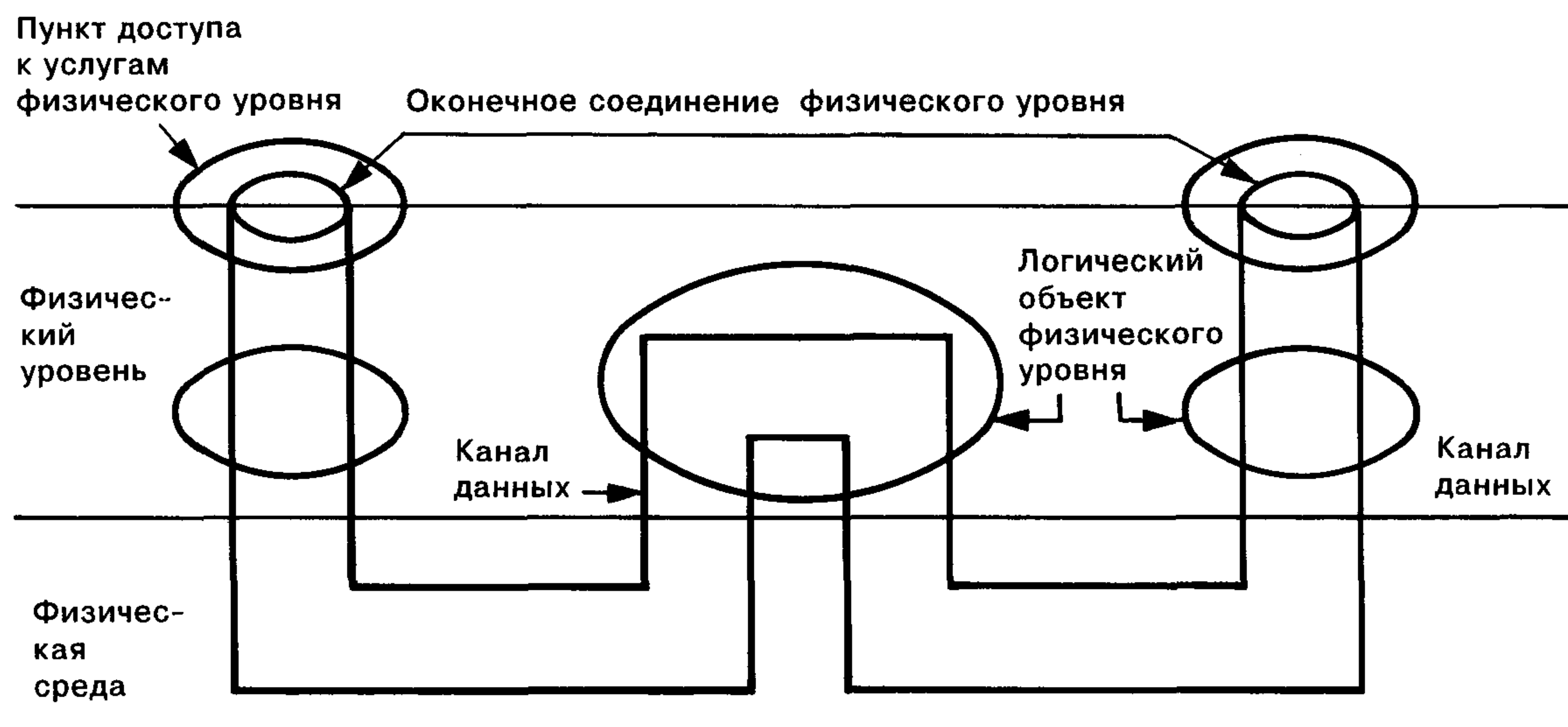
Рисунок 17 — Взаимосвязь каналов данных внутри физического уровня
