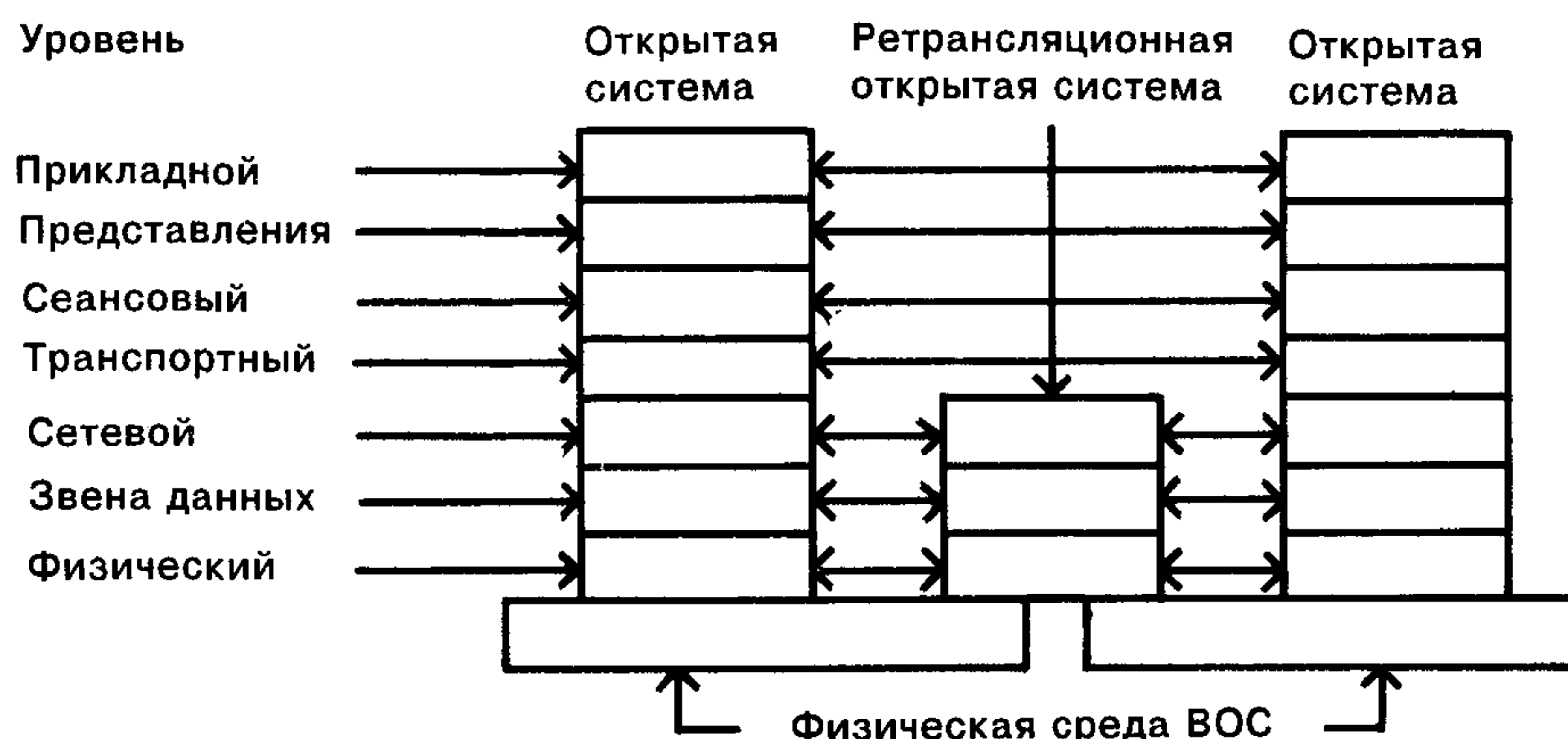
Рисунок 12 — Обмен данными через ретрансляционную открытую систему
