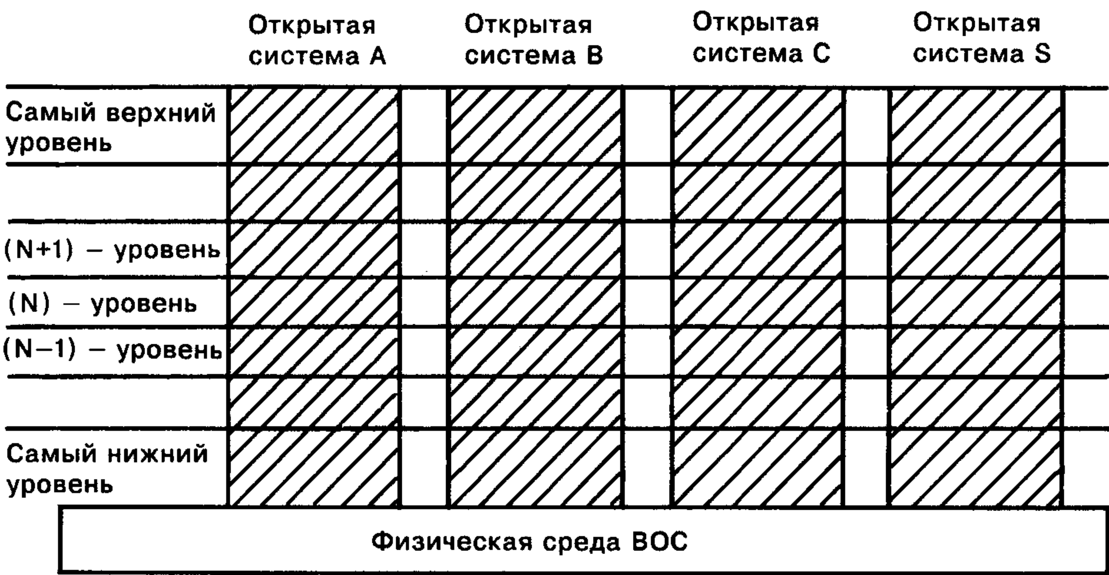
Рисунок 3 — Организация уровней во взаимосвязанных открытых системах
