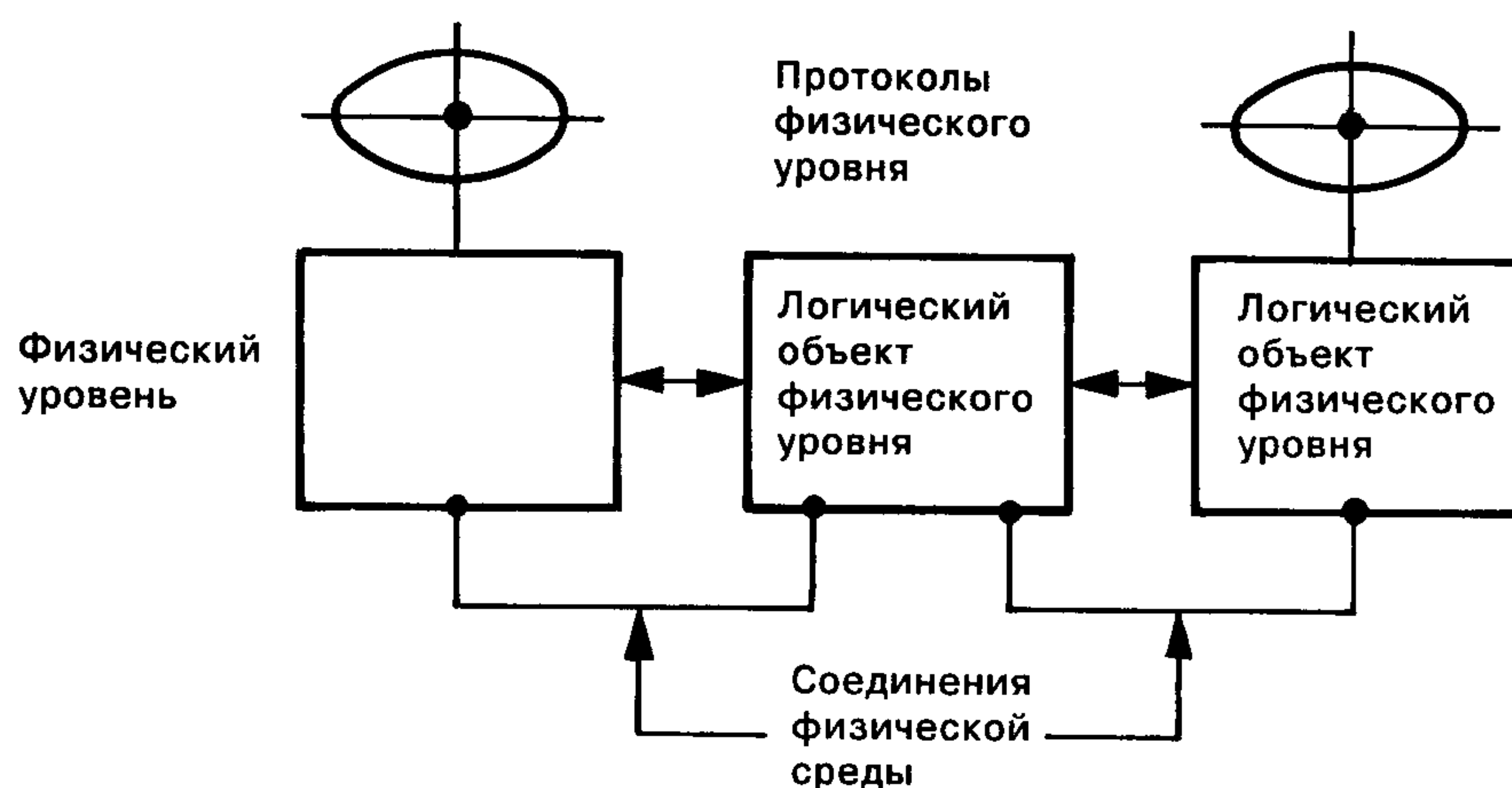
b) Логическая среда
