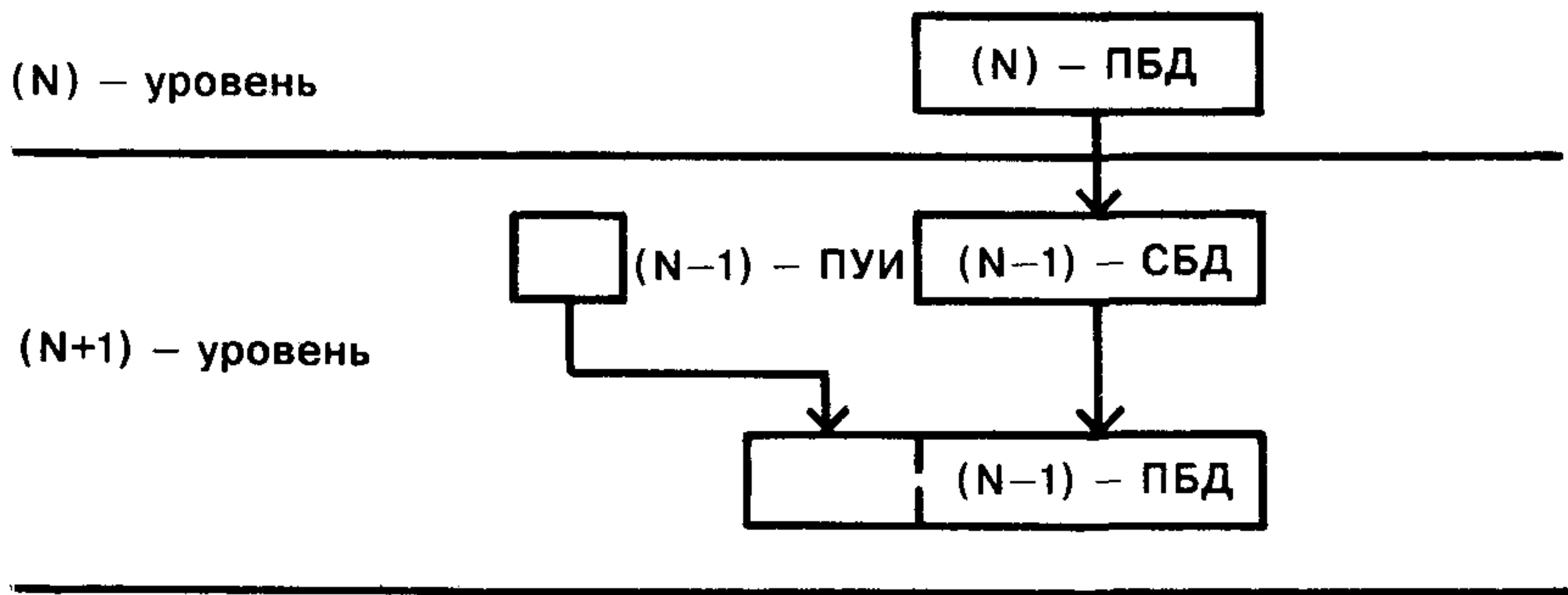
Рисунок 8 — Взаимоотношения между блоками данных
