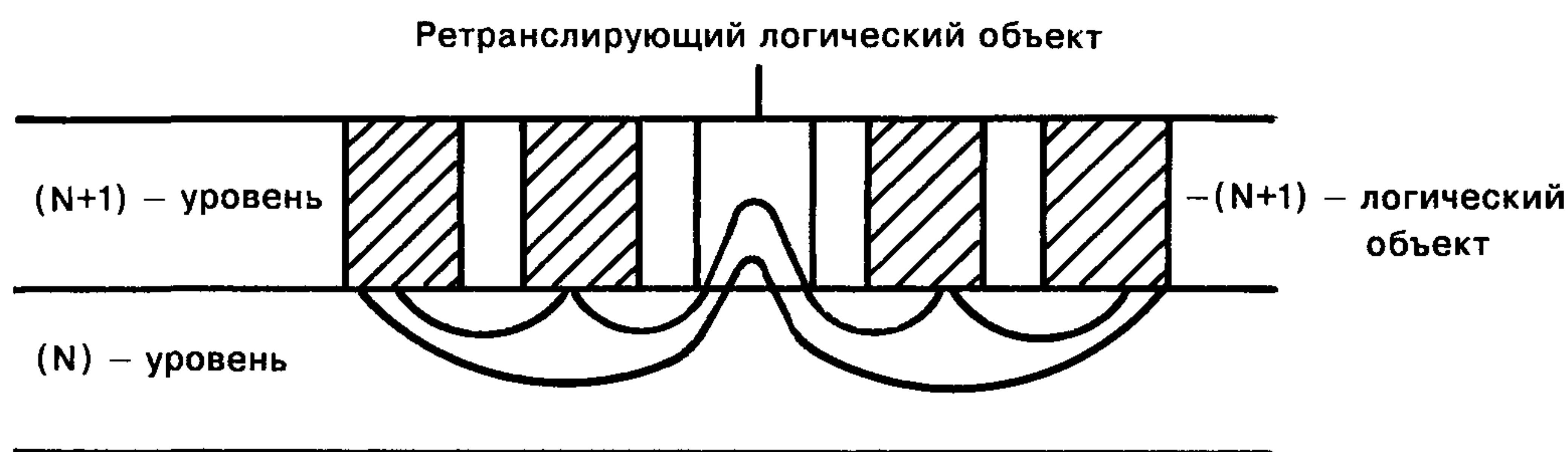
Рисунок 6 — Связь через ретранслятор
