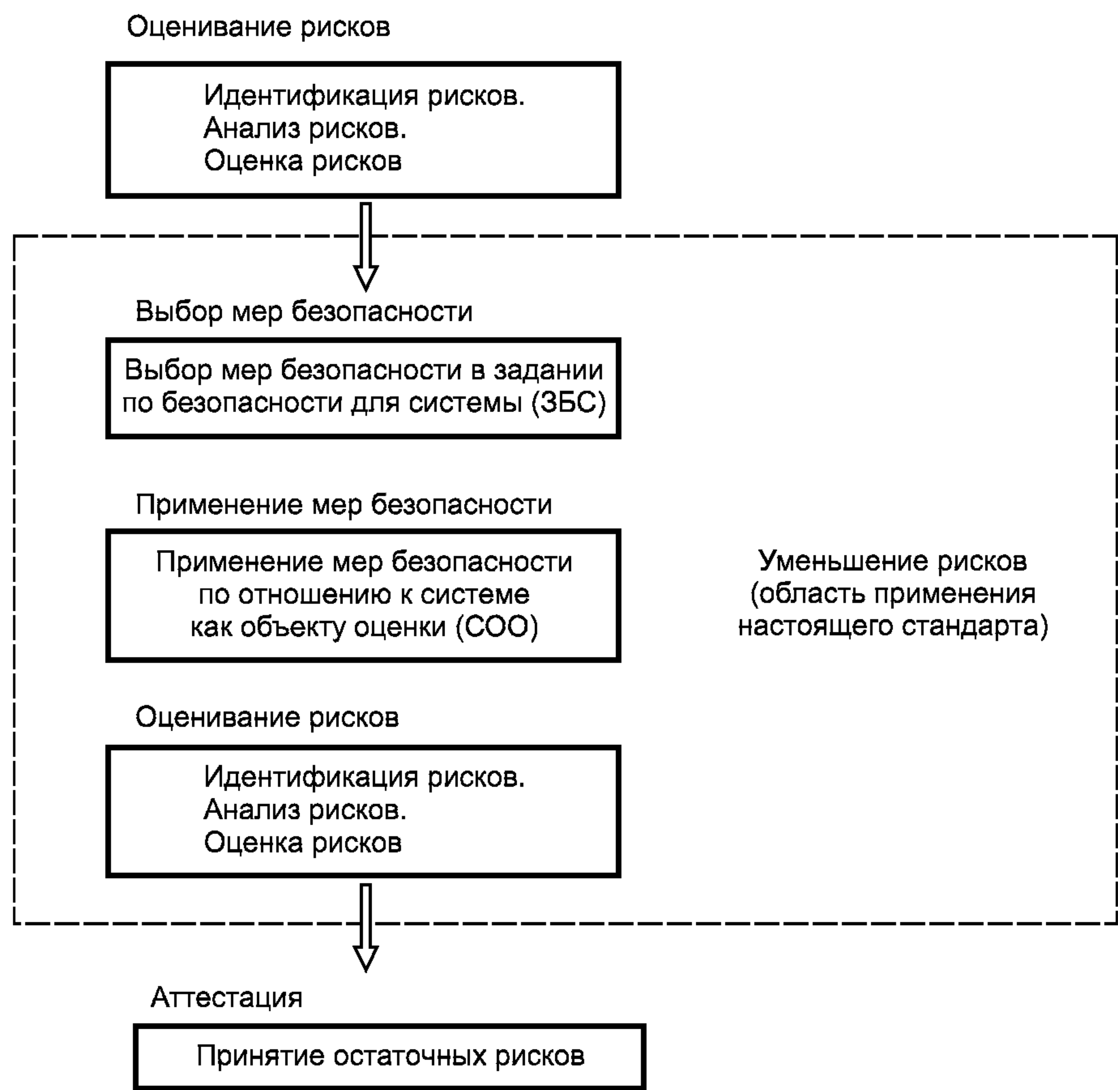
Рисунок 1 — Трехэтапный процесс обеспечения безопасности автоматизированных систем
